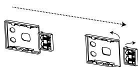
A. Бекіткіш рейкасының жапсырма қақпағын ажыратыңыз (№ 8)
