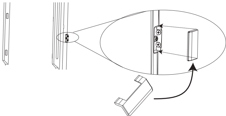
Установка декоративной накладки крепежного элемента (№ II)
