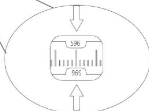
В. Вставьте рейку фиксатора в декоративную крышку рейки фиксатора (№ 8), переместите шкалу на отметку 596
