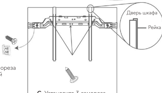
С. Установите 3 самореза по дереву (№ 22)
