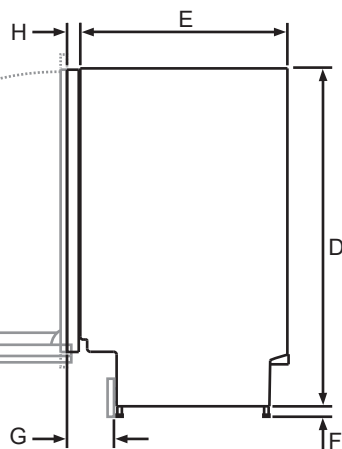
ВИД СБОКУ
