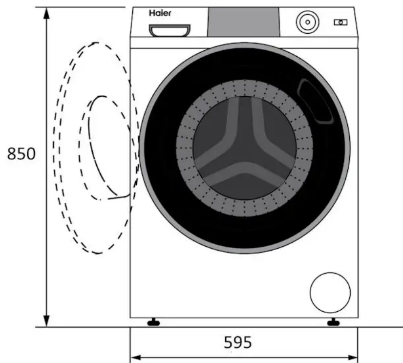
ВИД СПЕРЕДИ
